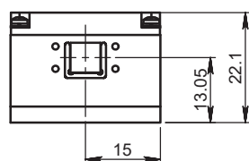
激光头尺寸图
