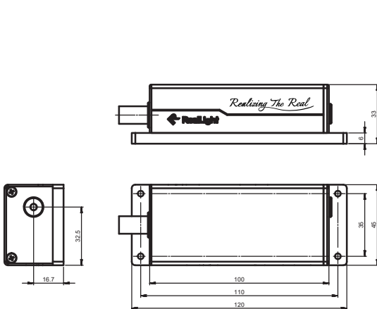
激光头尺寸图(侧出光)
