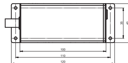
激光头尺寸图
