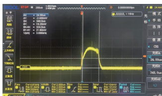
典型脉冲波形（2940nm）
