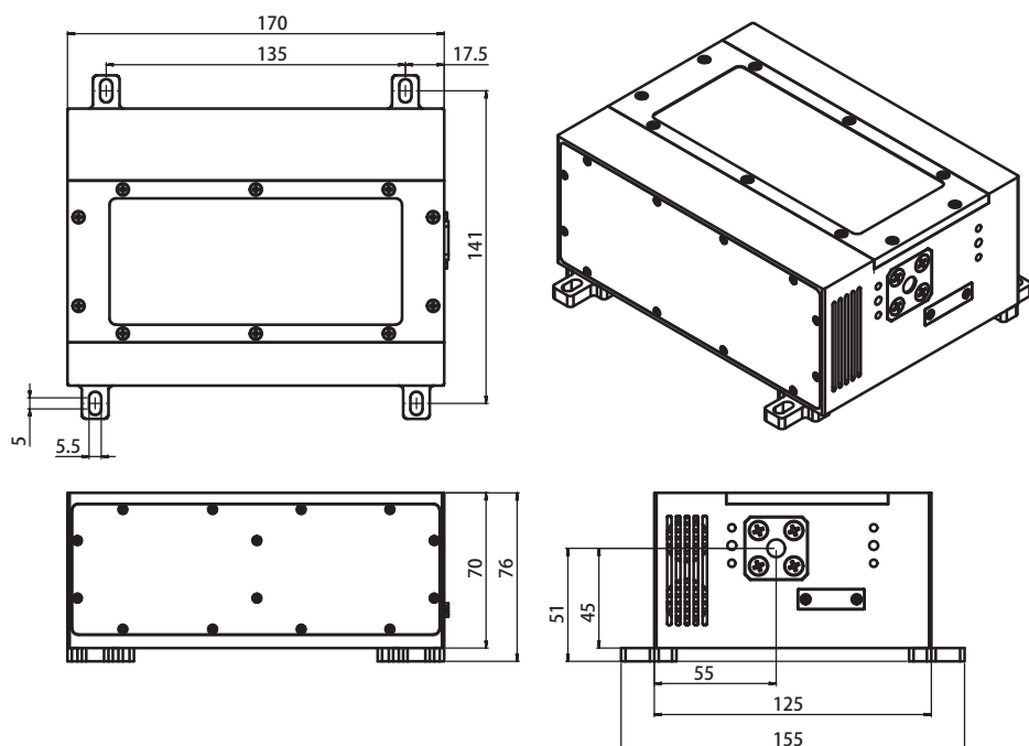
1064nm & 532nm 产品尺寸图
