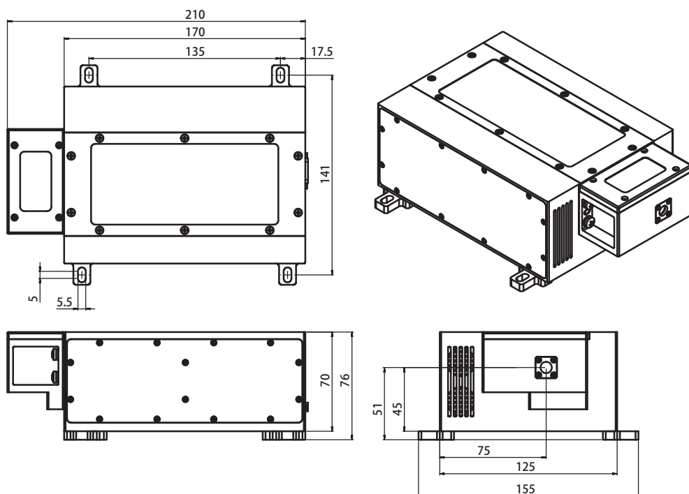
355nm & 266nm 产品尺寸图
