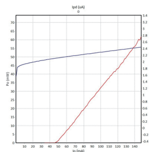
PIV曲线图
