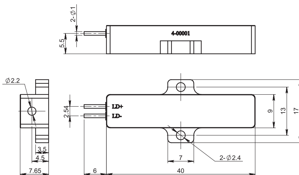
F4A尺寸图
