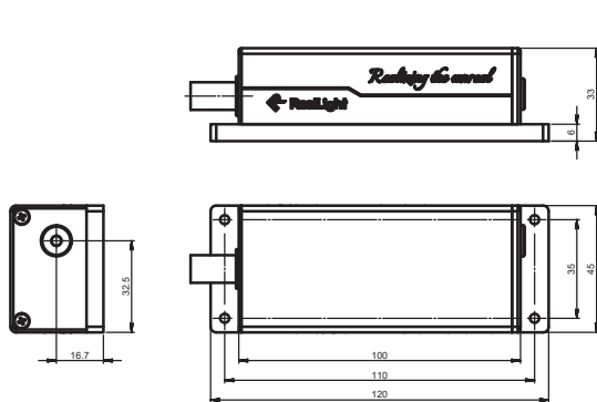
激光头尺寸图(侧出光)
