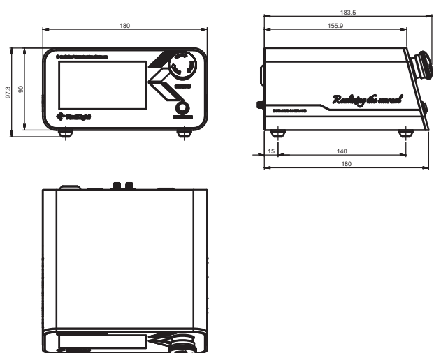
驱动电源尺寸图
