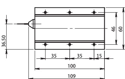
泵源尺寸图
